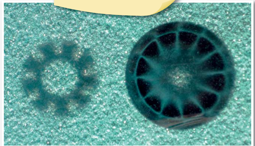
Erst die magnetische Detektorfolie lässt das Funktionsprinzip eines bürstenlosen Motors erkennen: Der Rotor enthält 12 unterschiedlich magnetisierte Bereiche, die ihn durch das Wechselfeld der 3 × 3 Magnetspulen in Drehung versetzen.
